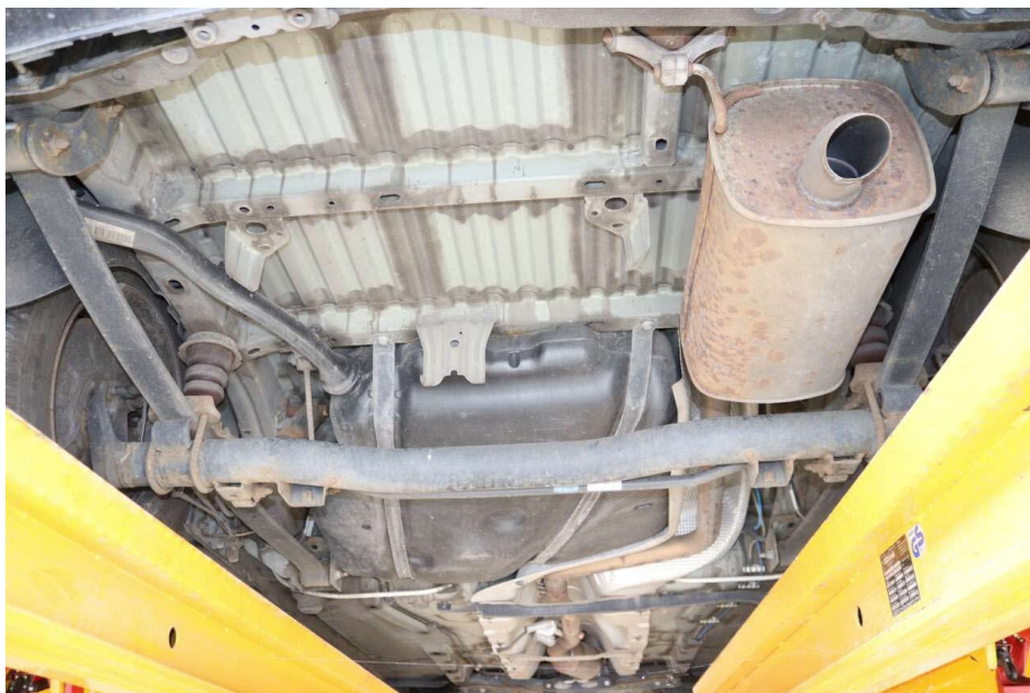
Bild 18 zeigt das Fahrzeug unterhalb von hinten
