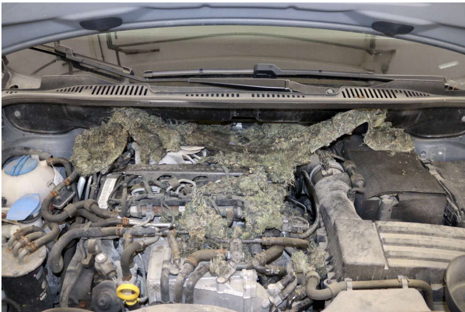
Bild 12 zeigt die beschädigte Motorraumdämmmatte
